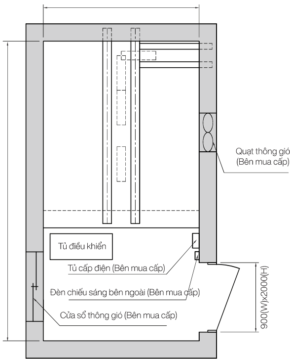
Mặt cắt ngang phòng máy
