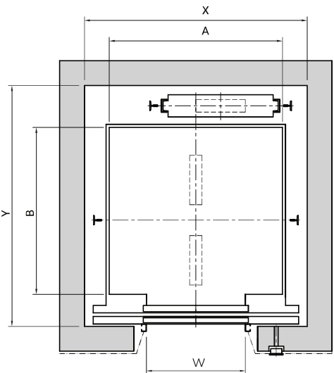
Mặt cắt ngang giếng thang
